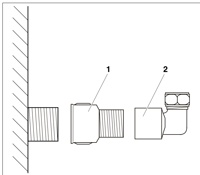
Obr. 4 Pripojenie k zásobníkom SM
